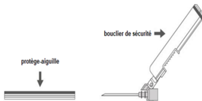
Figure C : Composants de l'aiguille de sécurité (préparés pour l'utilisation)
